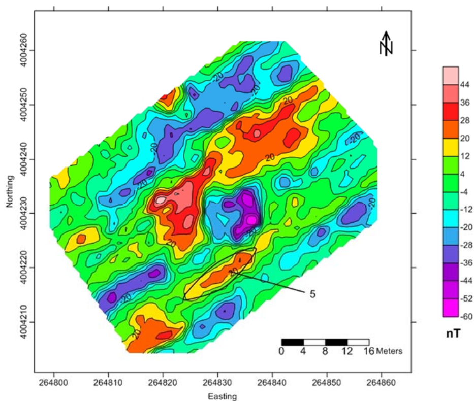
شکل ۸: بی‌هنجاری مغناطیسی باقیمانده از روند سطح مرتبه شش محدوده مورد مطالعه Fig. 8: Residual magnetic anomaly from 6 th order trend surface method on the study area
