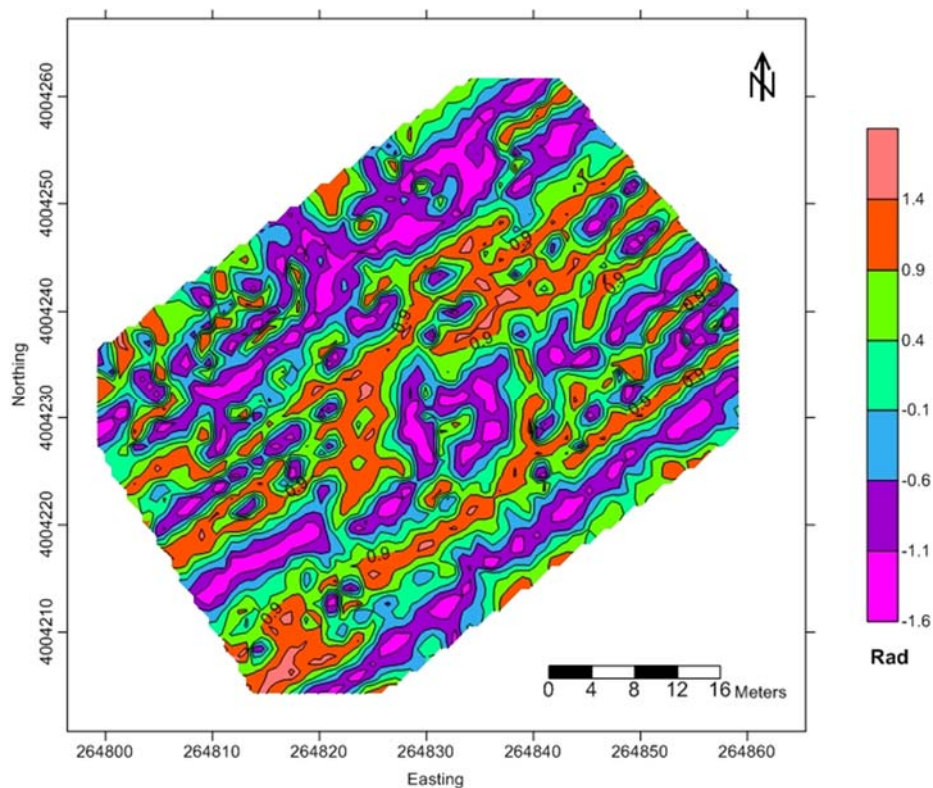
شکل ۹: نقشه اعمال فیلتر زاویه تمایل روی بی‌هنجاری مغناطیسی محدوده مورد مطالعه Fig. 9: Tilt angle map of magnetic data covering study area, Tepe Hissar
