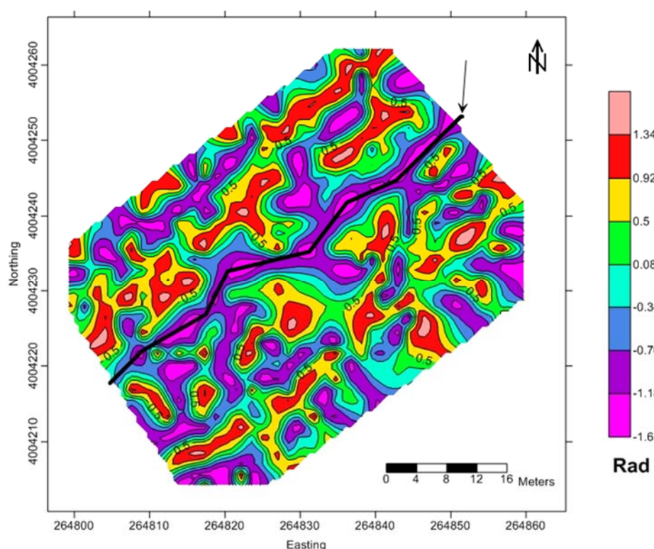
شکل ۵: نقشه اعمال فیلتر زاویه تمایل روی بی‌هنجاری گرانی محدوده مورد مطالعه
